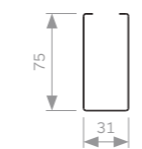
Sección lama (cotas en mm)
