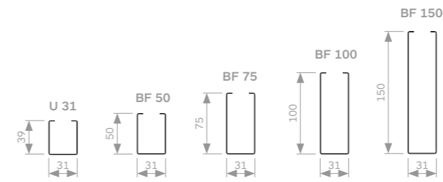
Sección lama (cotas en mm)
