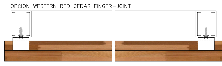
Planta E: 1/4
