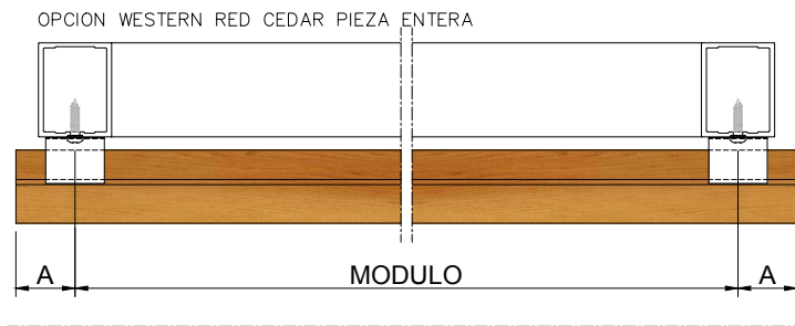
Alzado E: 1/4
